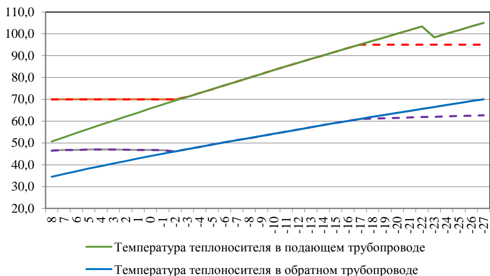
Рисунок 16 – Предлагаемый схемой теплоснабжения температурный график
