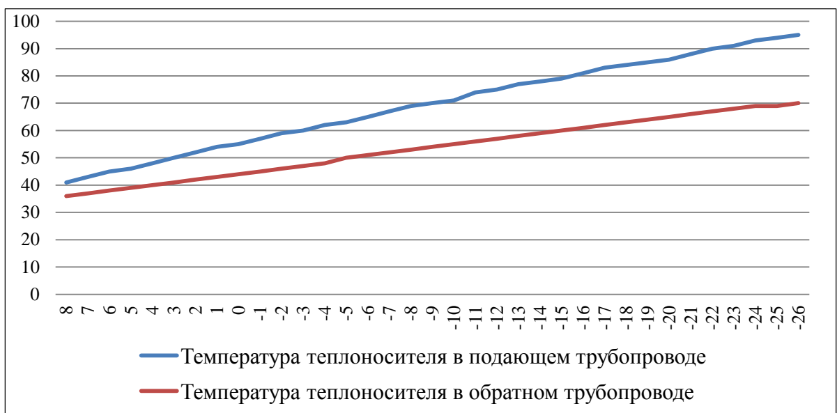
Рисунок 11 – Температурный график отпуски тепловой энергии от котельных ДРСУ, ДДИ, ул. Цветкова и ул. Заозерная
