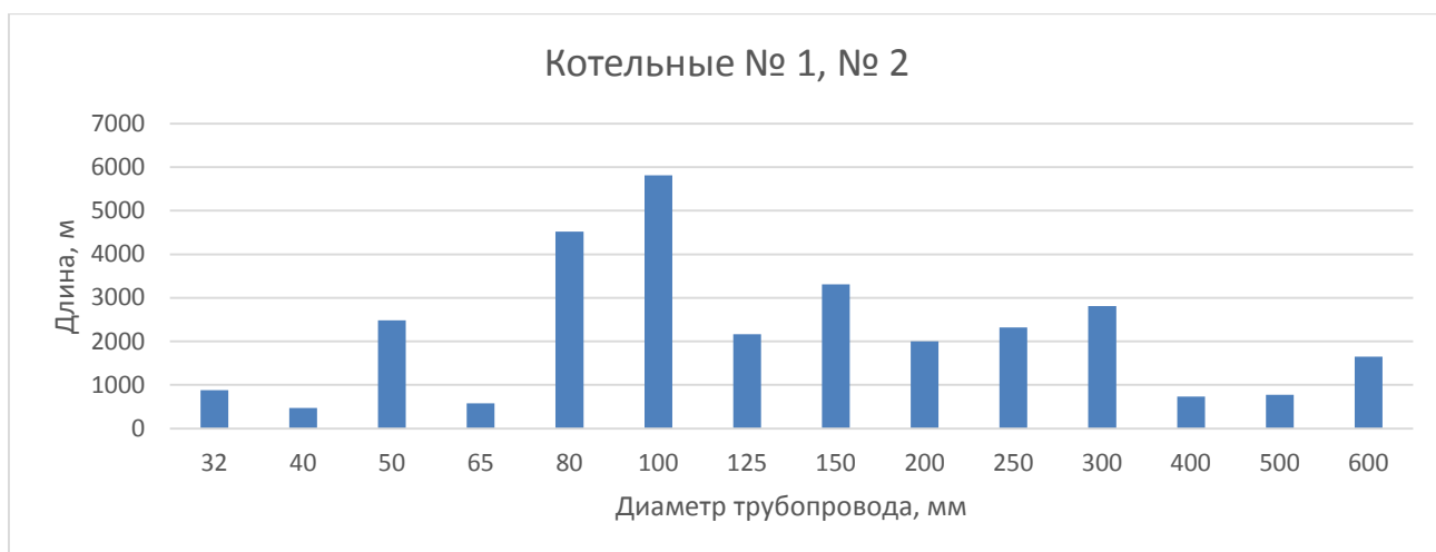
Рисунок 4 – Структура тепловых сетей от котельных №1, № 2
