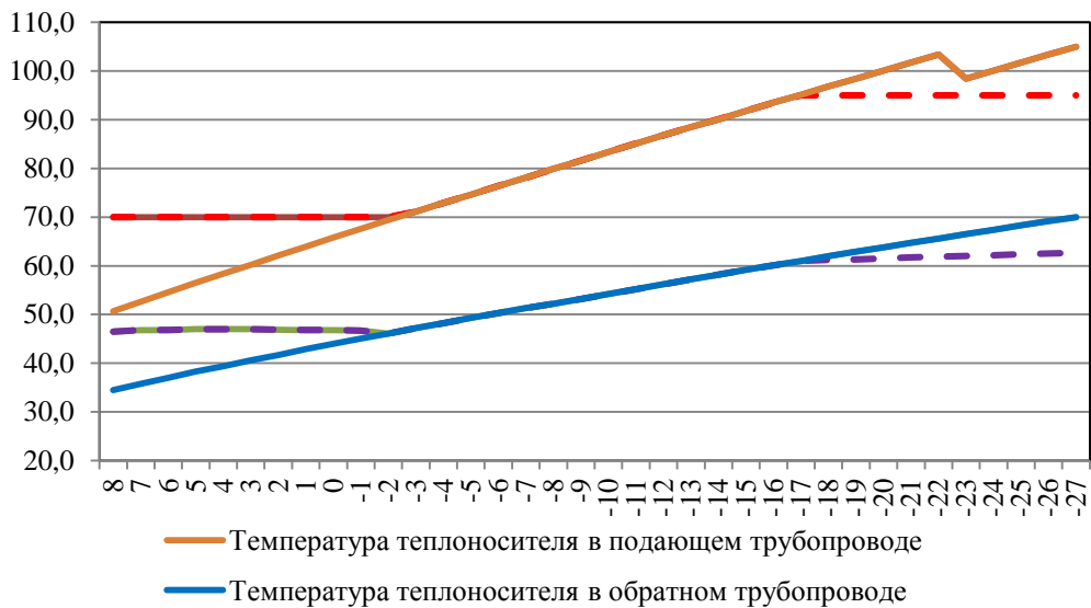
Рисунок 10 – Температурный график отпуски тепловой энергии от котельных № 1, № 2
